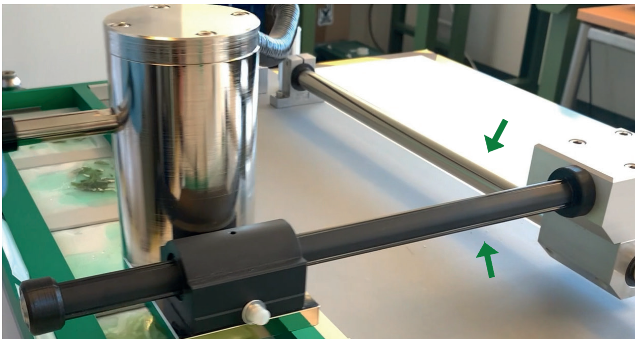
Abb. 1 Gleitachsen
